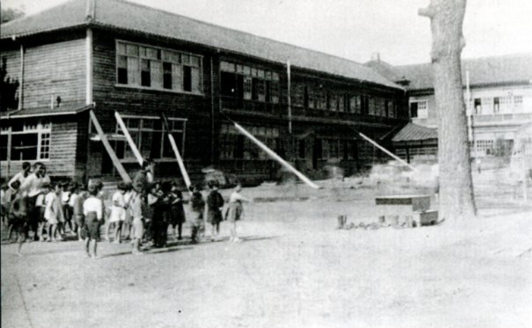
つかい棒で補強された地震後の鳥取師範附属小学校
