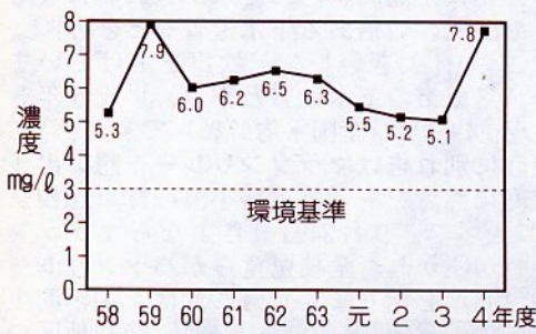
湖山池のCODの経年変化
