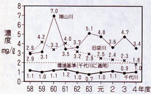
各河川のBODの経年変化
