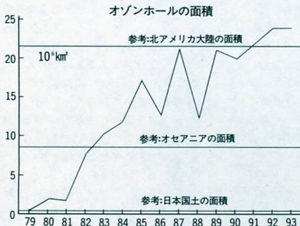
南極のオゾンホールの変化
