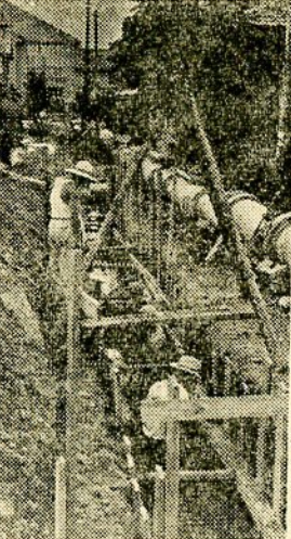
寺町の下水道布設工事
