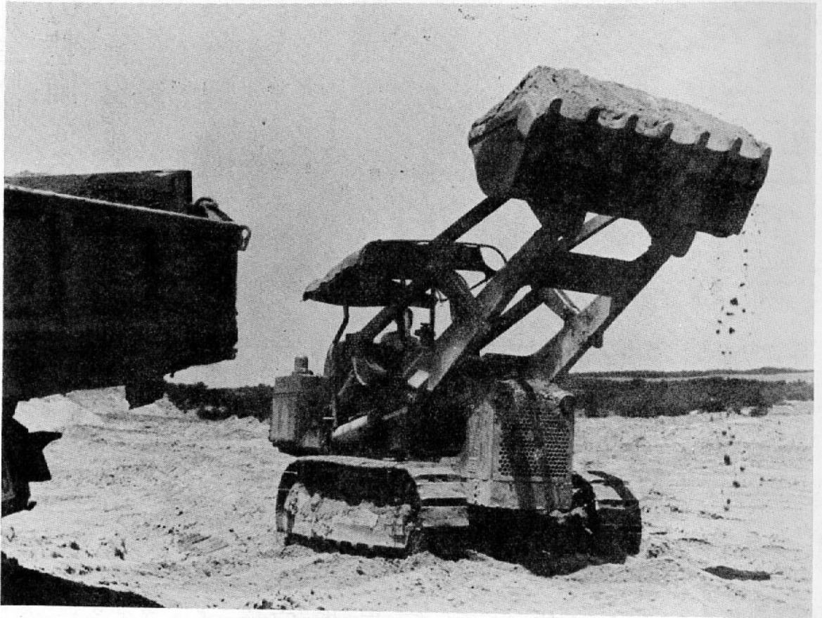
住宅団地の造成に活躍するドーザーシャベル (湖山地区)
