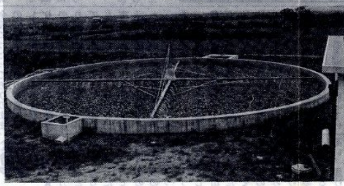
↑ 散水ろ床 深さ1.9に50ミリ~60ミリ級の碎石を敷きならべたろ床に下水を連続散水する。ろ材の表面にできるろ模の働き、すなわち、表面に生息する種々の好気性微生物の働きによって、下水道のなかの有機物や溶存物質が酸化分解して無機物となり、浄化される。
