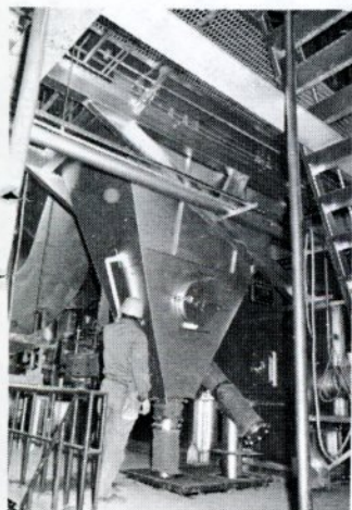
排ガス中のダストを捕集するマルチサイクロン集塵装置
