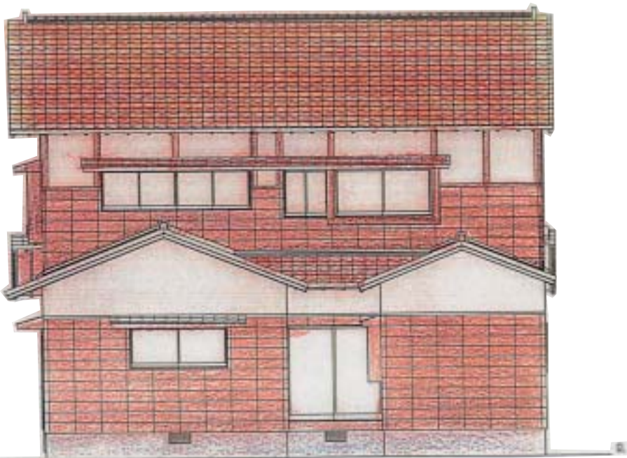
北側立面図 1/100
