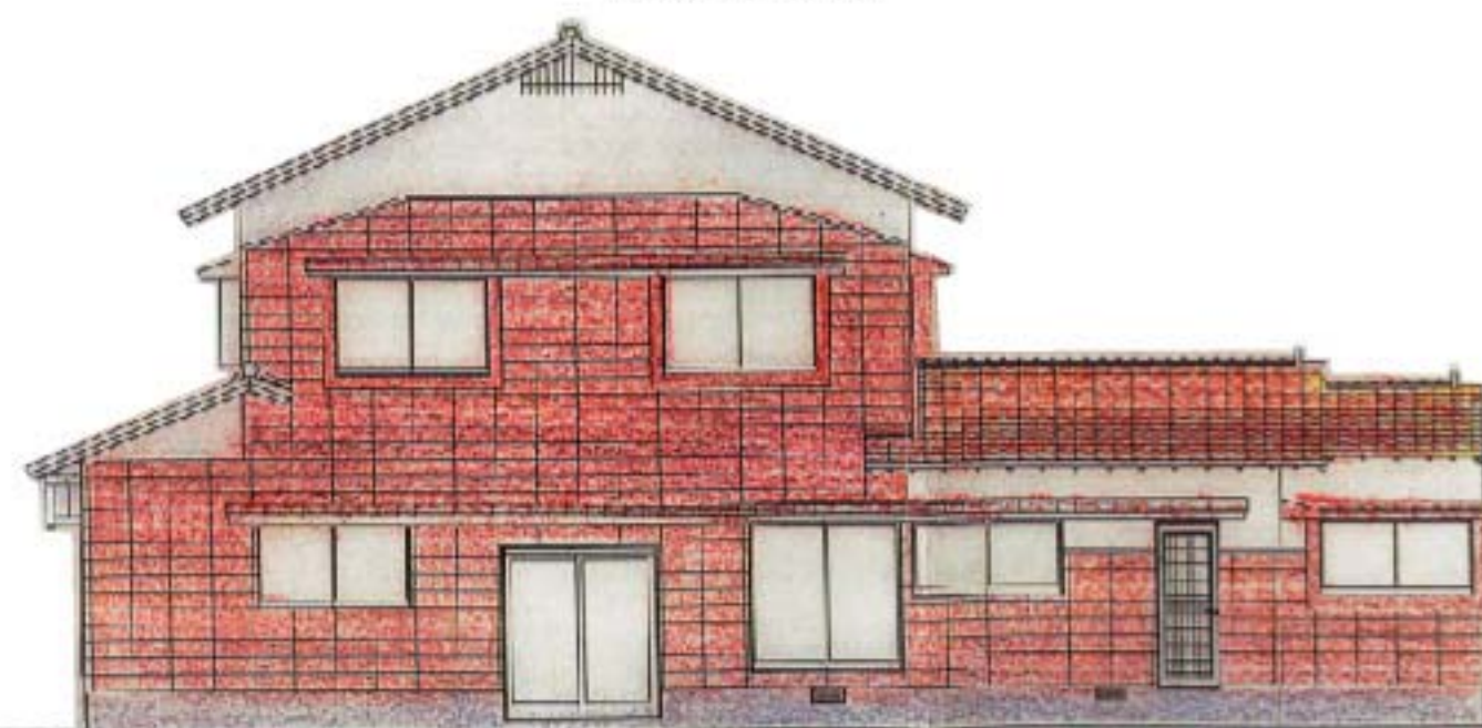
東側立面図 1/100
