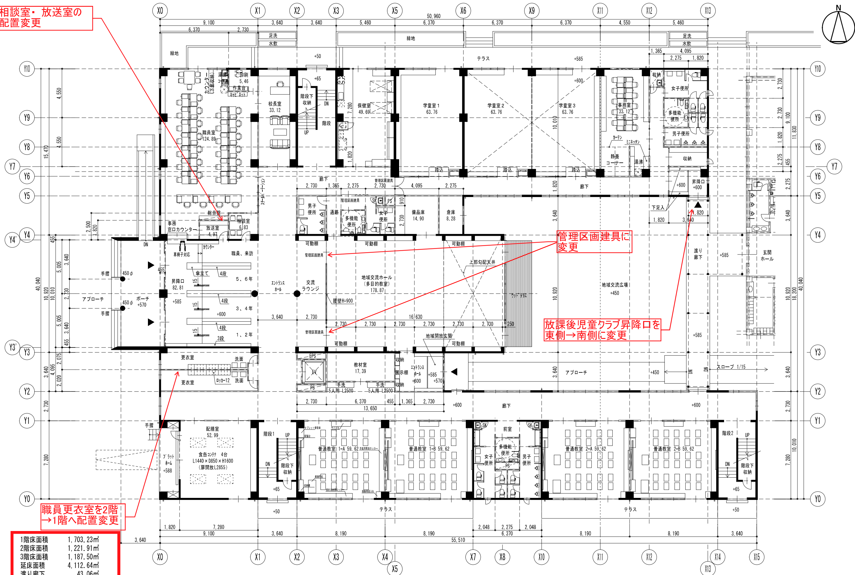
1階平面図
