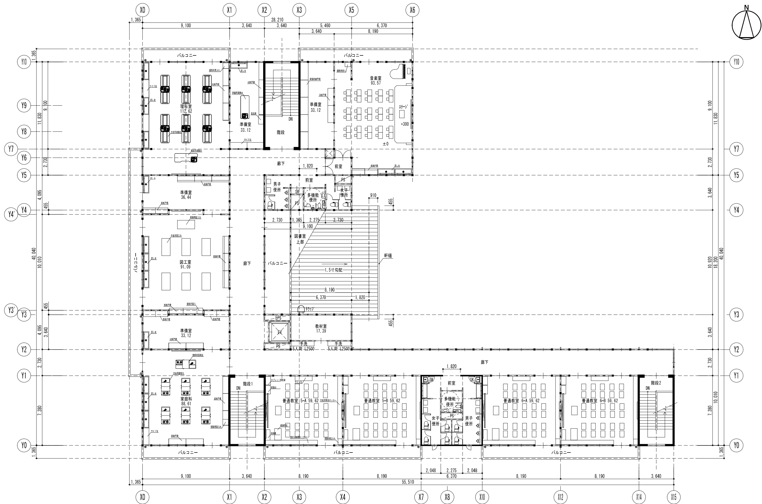
3階平面図 S = 1:200
