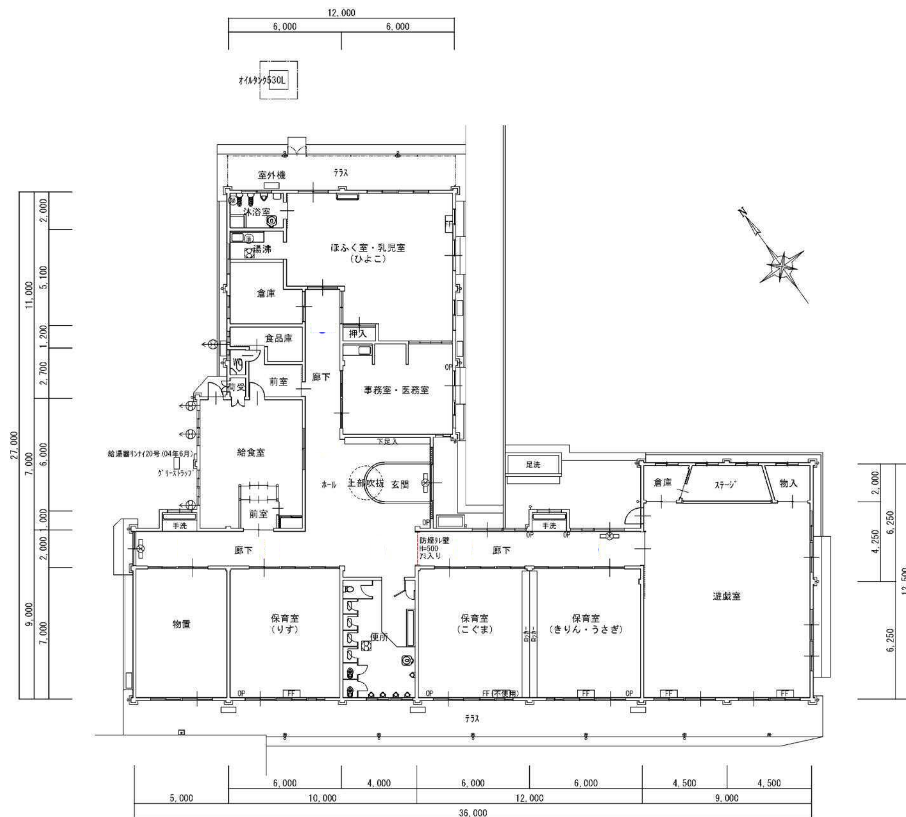
1 階平面図 1/200
