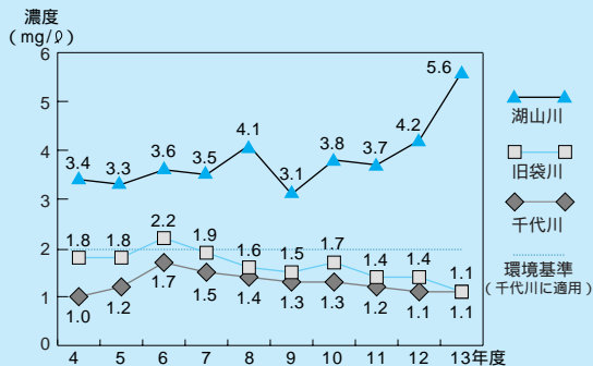
～ 各河川のBODの経年変化～
