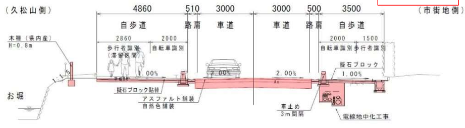
標準横断面
