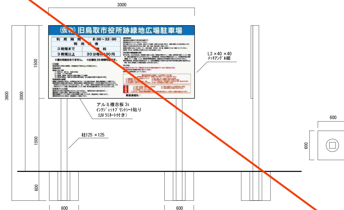
自立料金規約看板 S=1:40
