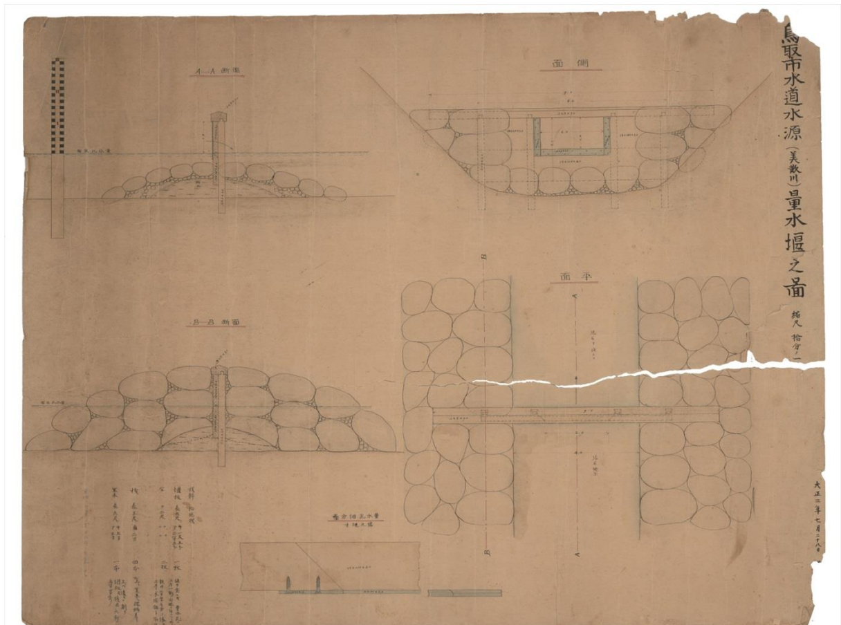
No-64 鳥取市水道水源量水堰之図
