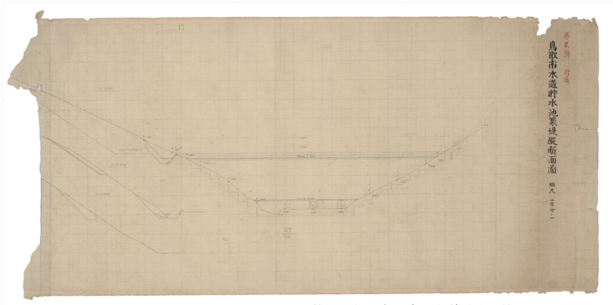
No-28 第二号付属鳥取市上水道貯水池築堤断面図
