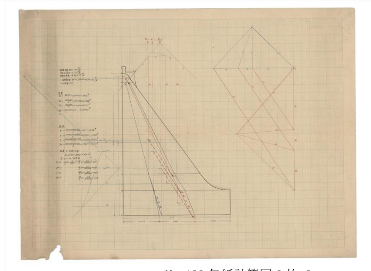
No-139 包紙計算図 2 枚-2
