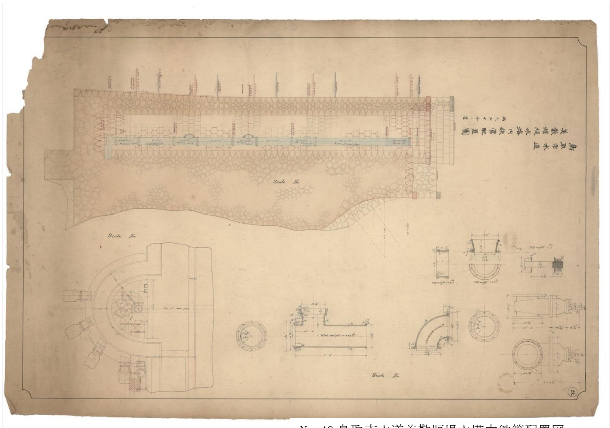
No-49 鳥取市水道美敷堰堤水塔内鉄管配置図
