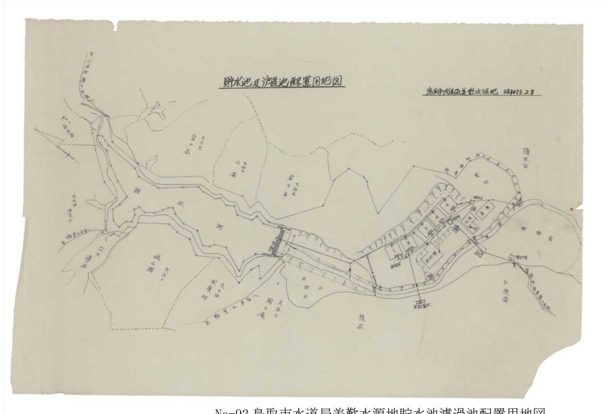
No-92 鳥取市水道局美敷水源地貯水池濾過池配置用地図
