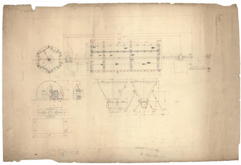
No-76 砂洗機原図
