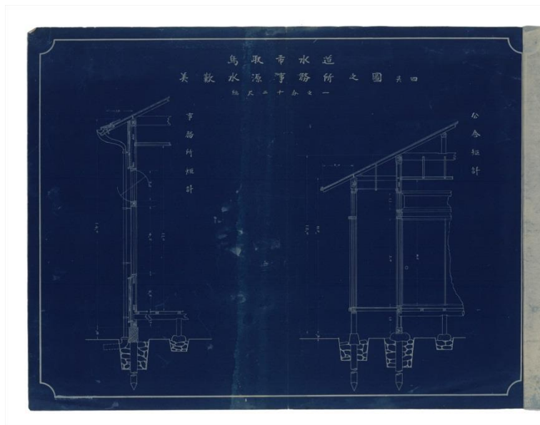
No-16 美歎水源事務所之図-5
