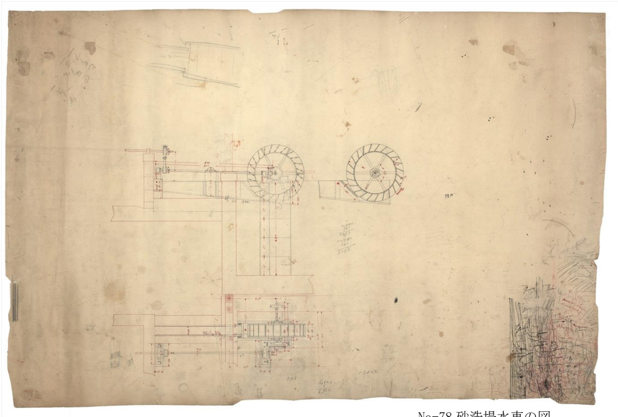
No-78 砂洗場水車の図
