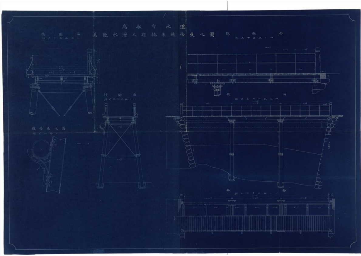
No-14 鳥取市水道美歎水源人道橋兼鉄管受之図
