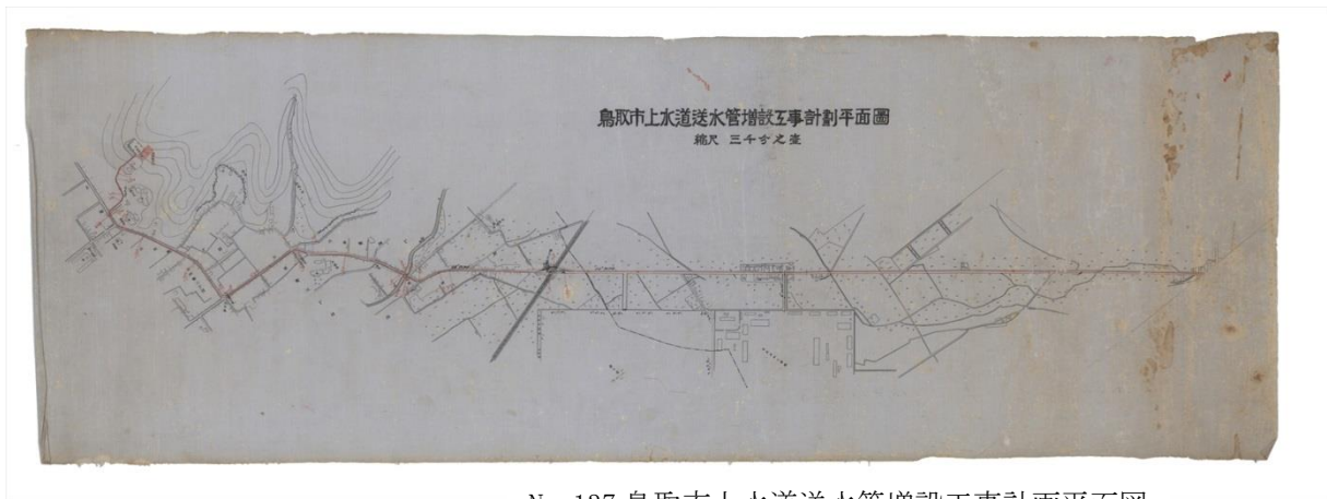
No-137 鳥取市上水道送水管増設工事計画平面図
