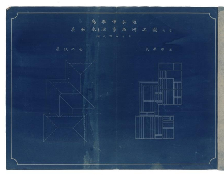
No-16 美歎水源事務所之図-4
