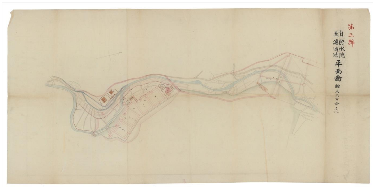
No-95 第三号自貯水池至濾過池平面図
