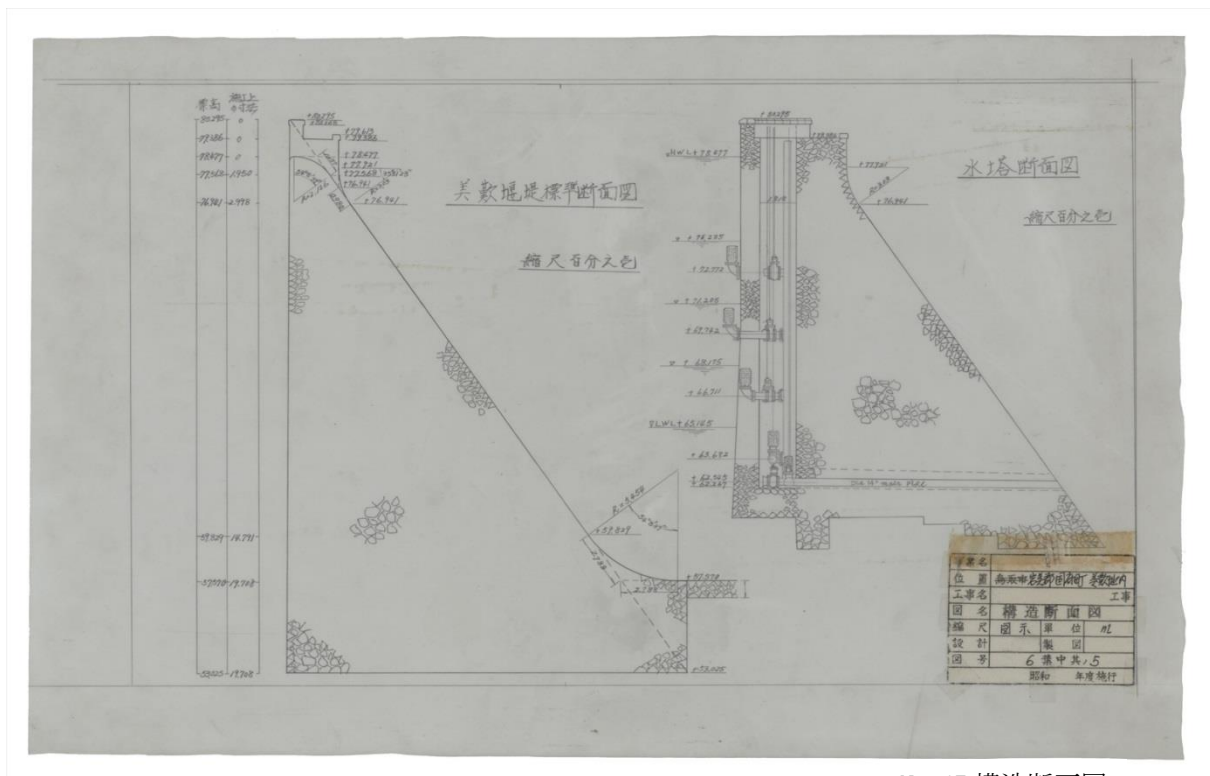
No-47 構造断面図
