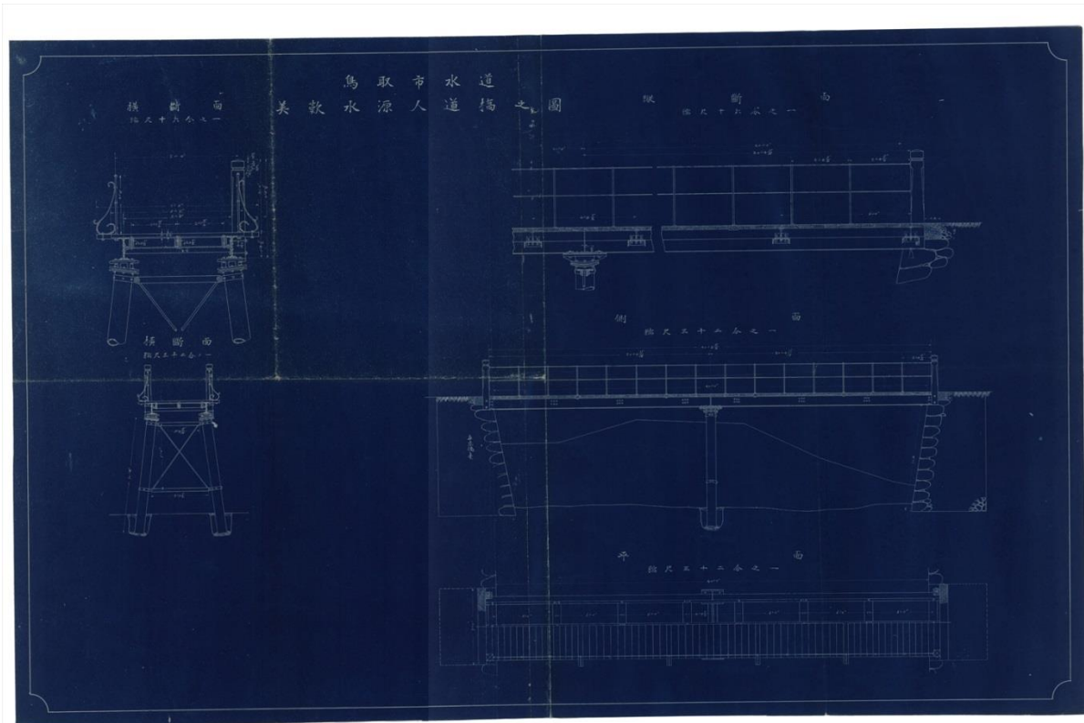
No-13 鳥取市水道美歎水源人道橋之図
