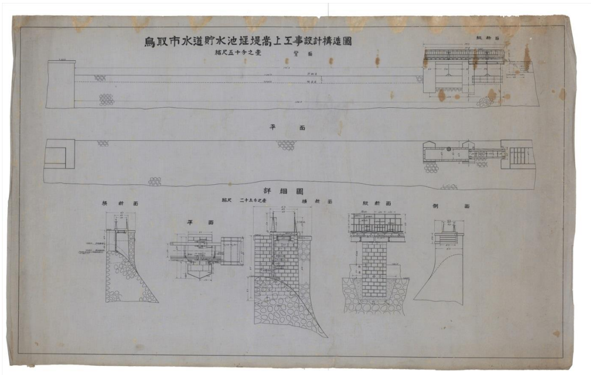
No-31 鳥取市水道貯水池堰堤工事設計構造図
