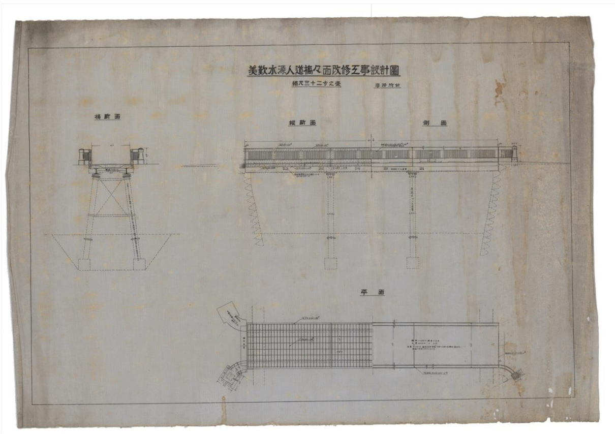
No-82 美敷水源人道橋々面改修工事設計図事務所前
