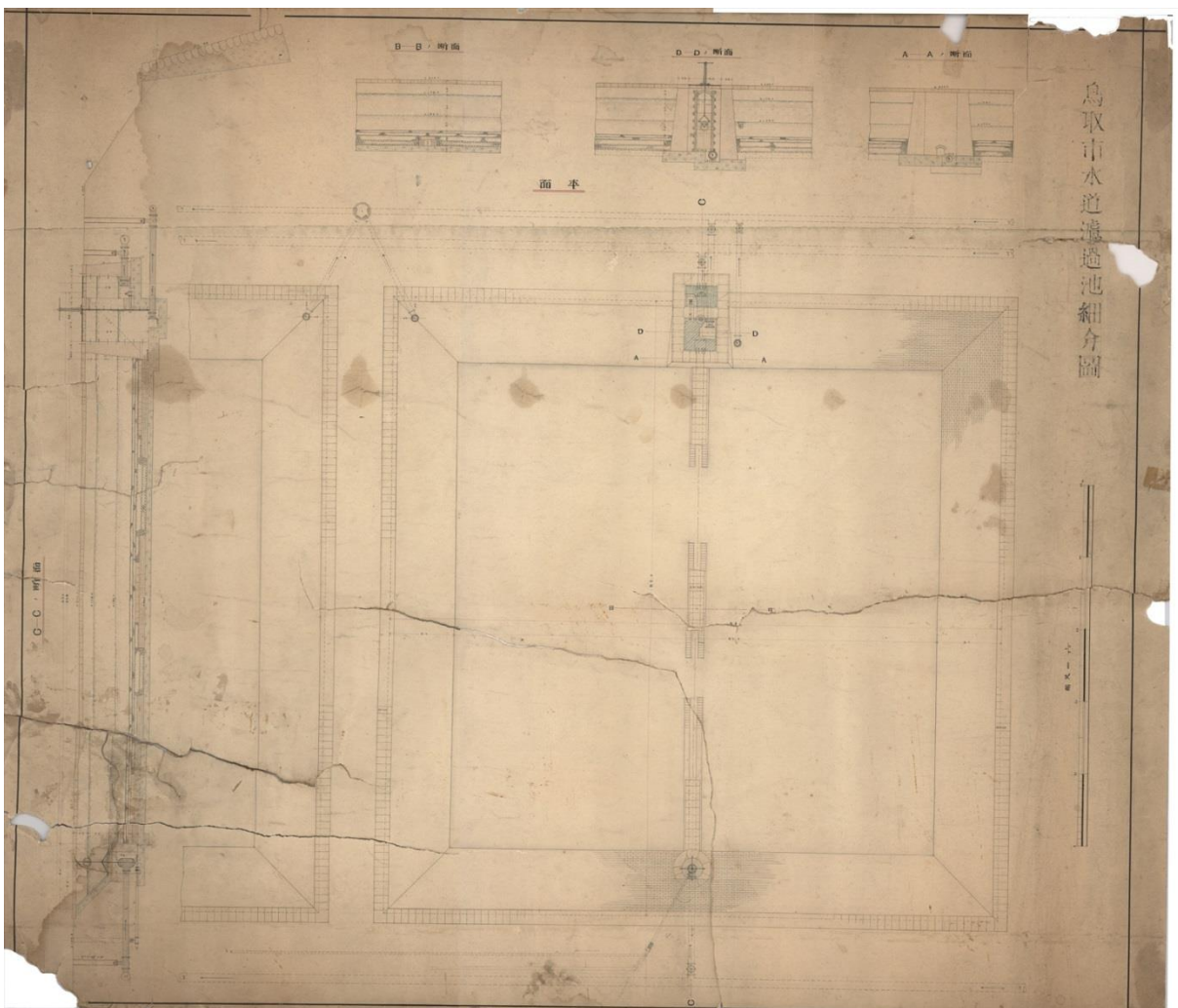
No-73 鳥取市水道濾過池細分図
