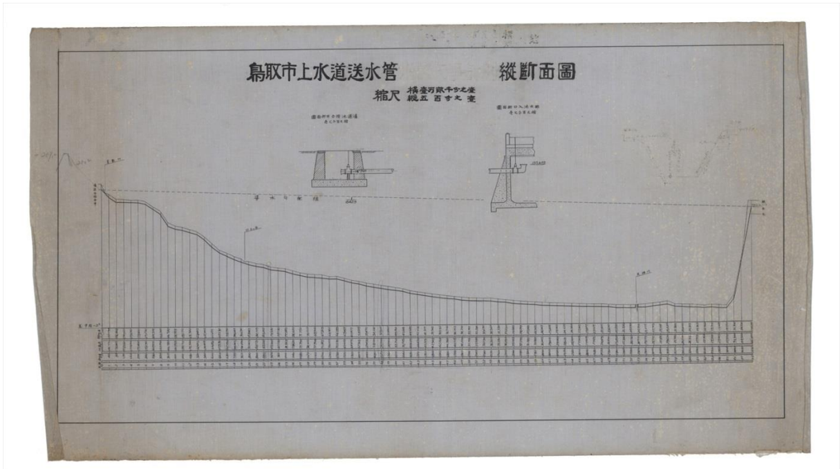
No-133 鳥取市上水道送水管増設工事計画縦断面図
