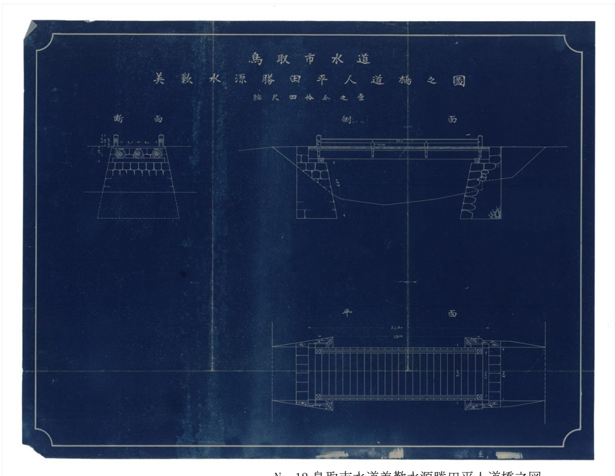
No-12 鳥取市水道美歎水源勝田平人道橋之図
