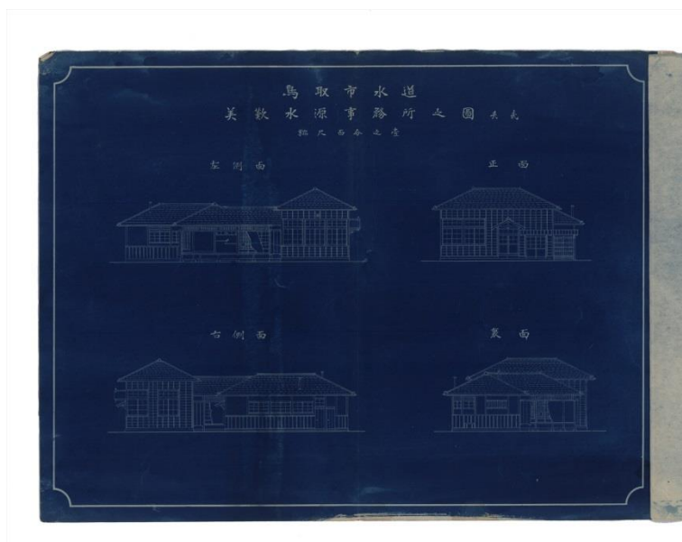
No-16 美敷水源事務所之図-3
