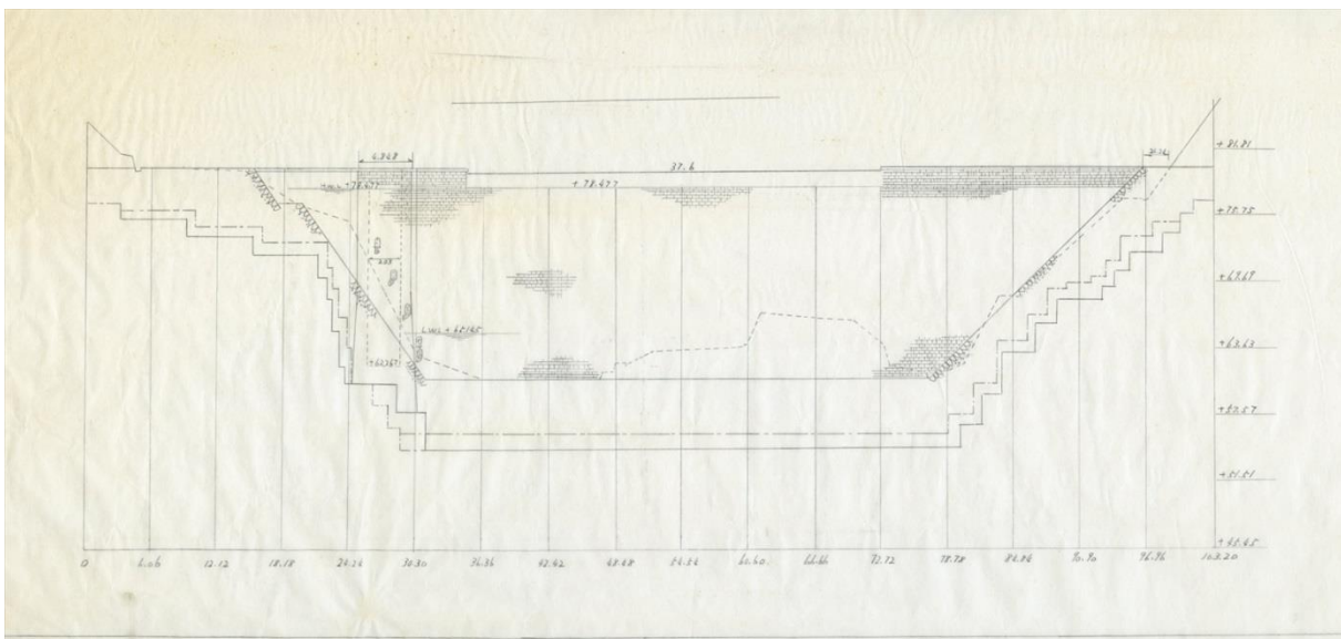
No-38 美歎堰堤正面図
