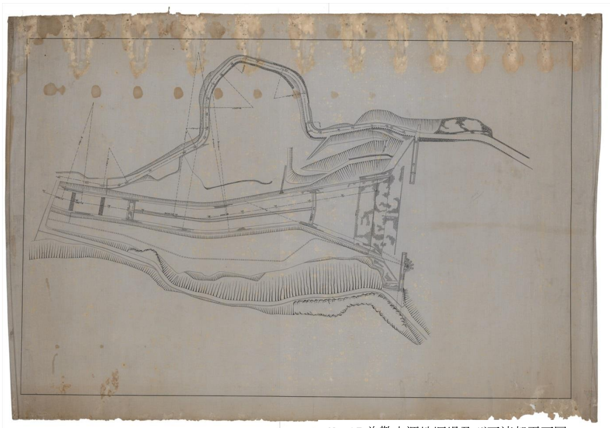
No-37 美歎水源地堰堤及び下流部平面図
