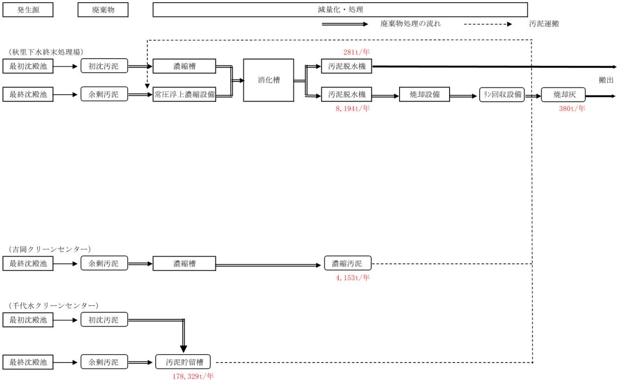
廃棄物処理フローシート
