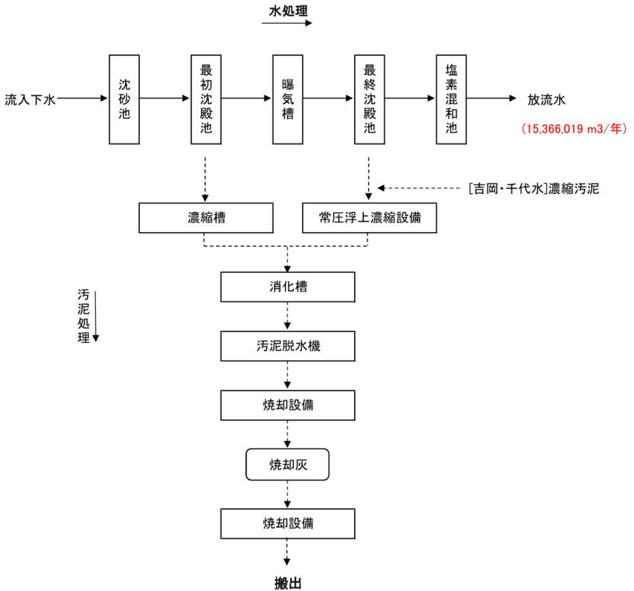
秋里下水終末処理場 処理フローシート
