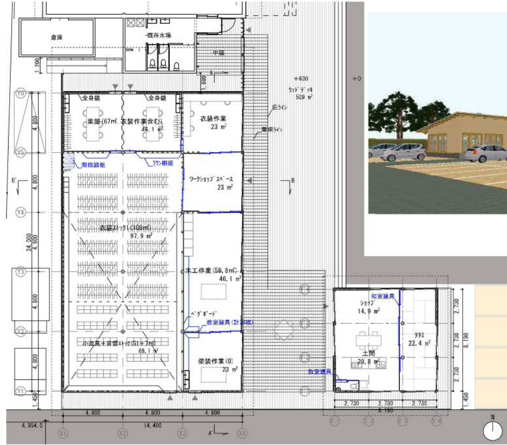
1階平面図 1:200
