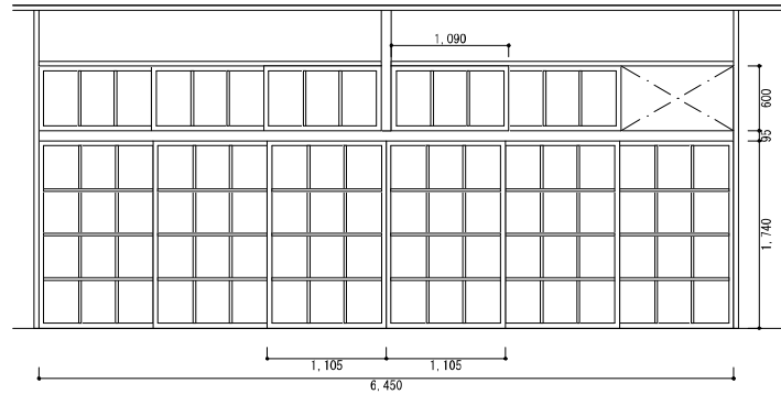
家庭科室 建具実測図面 1:50
