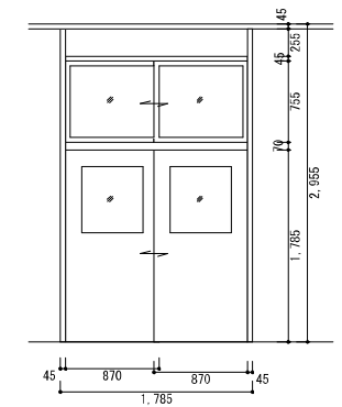
教室木製建具実測図面 1:50
