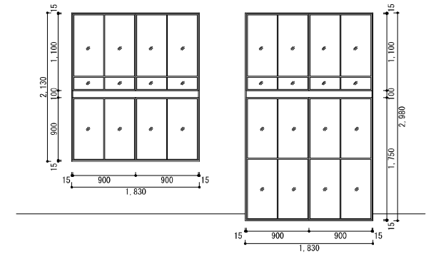
スチールサッシ実測図面 1:50
