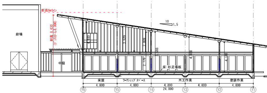
A-A' 断面図 1:200
