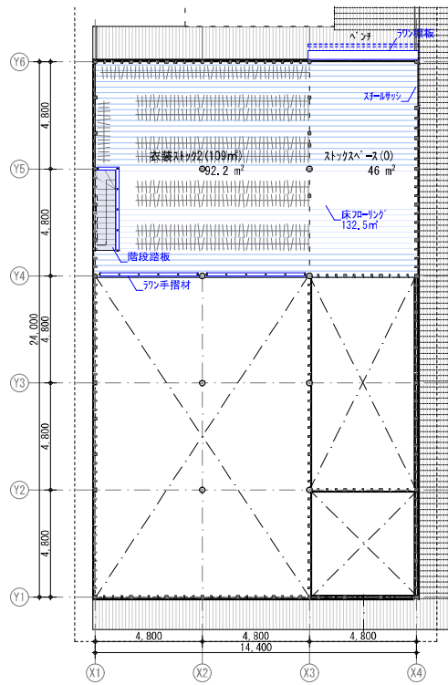
2階平面図 1:200
