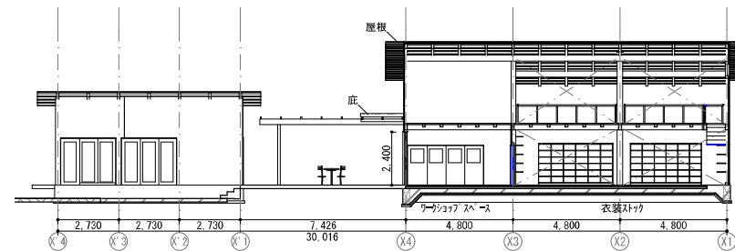
B-B' 断面図 1:200
