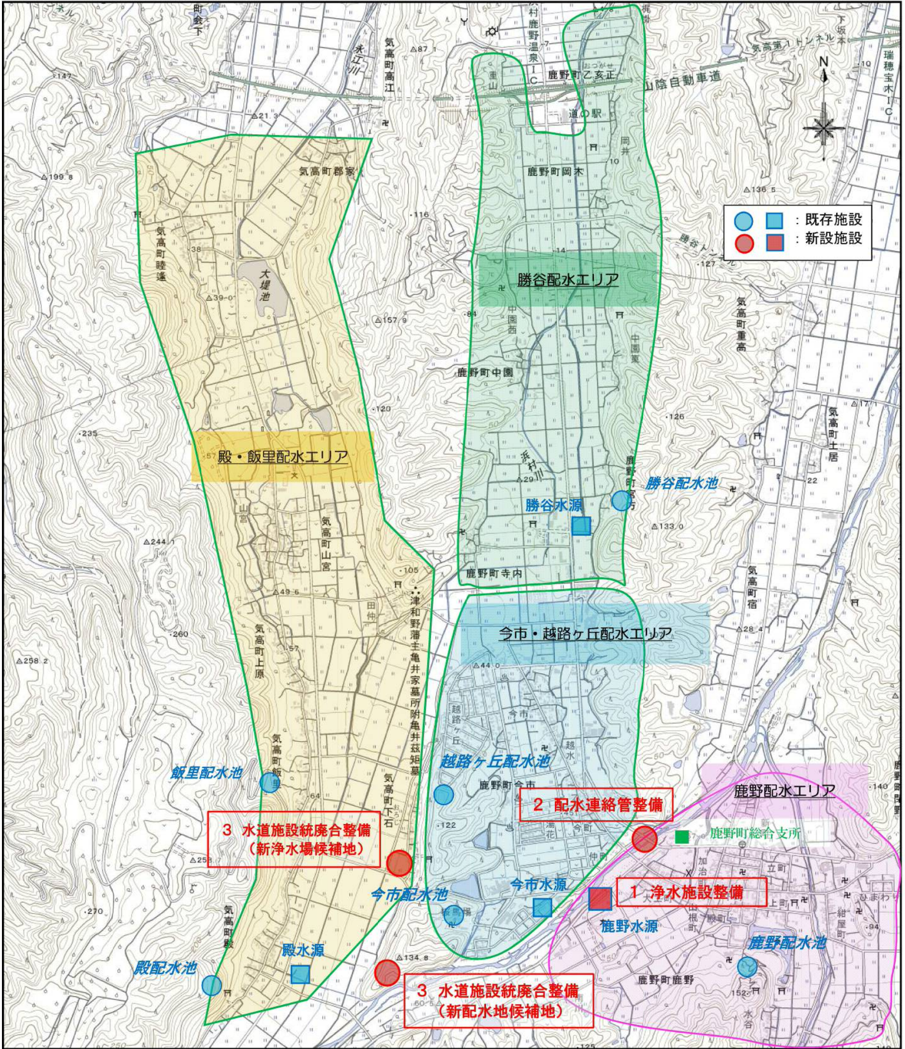
水道施設整備計画位置図
