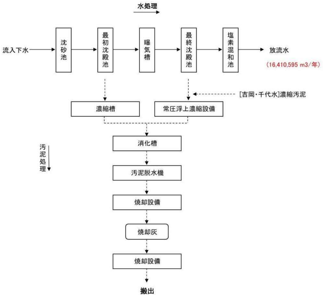
秋里下水終末処理場 処理フローシート
