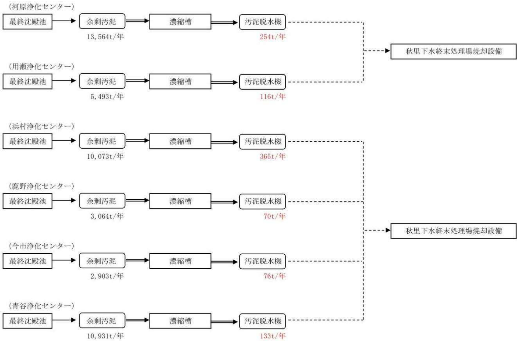
廃棄物処理フローシート
