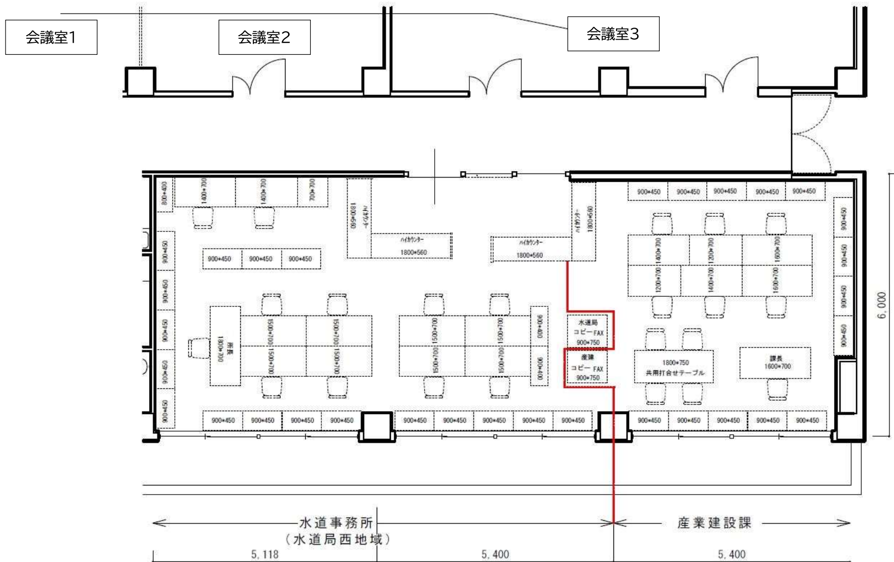
B棟2階 既存床の上に転がし配線
