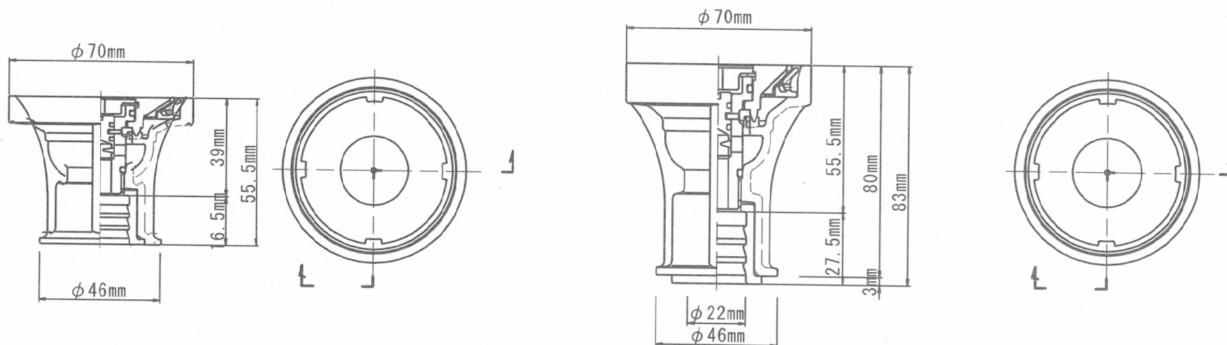
消雪散水ノズル仕様
