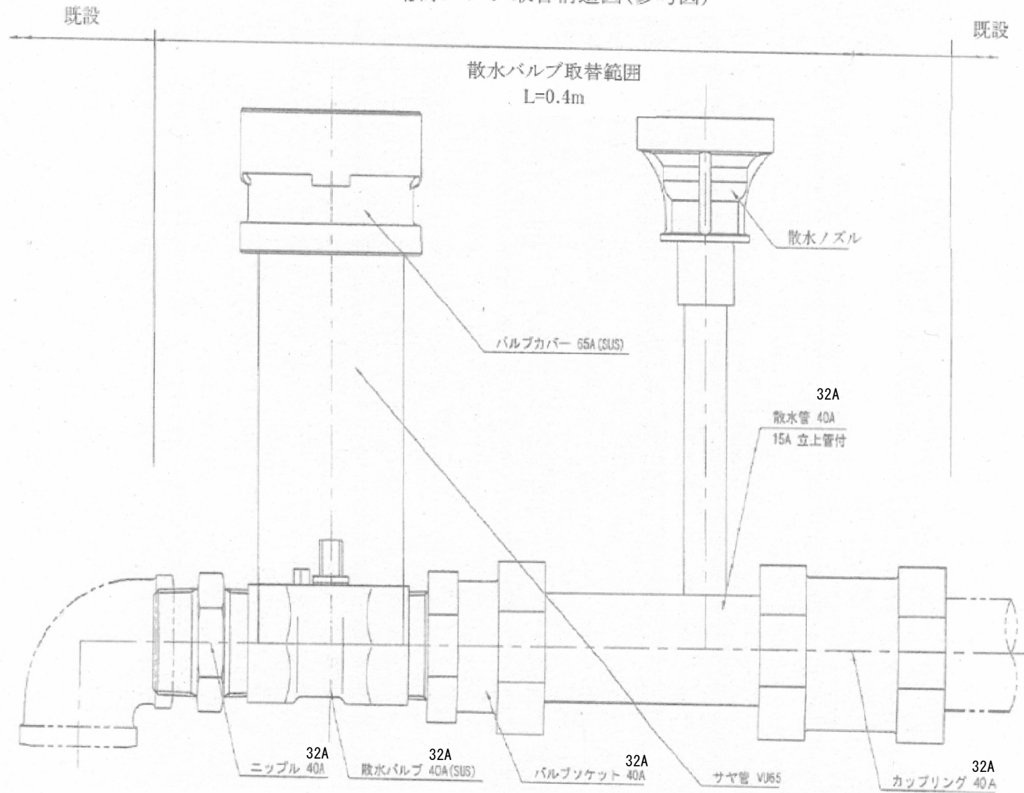
散水バルブ取替構造図(参考図)
